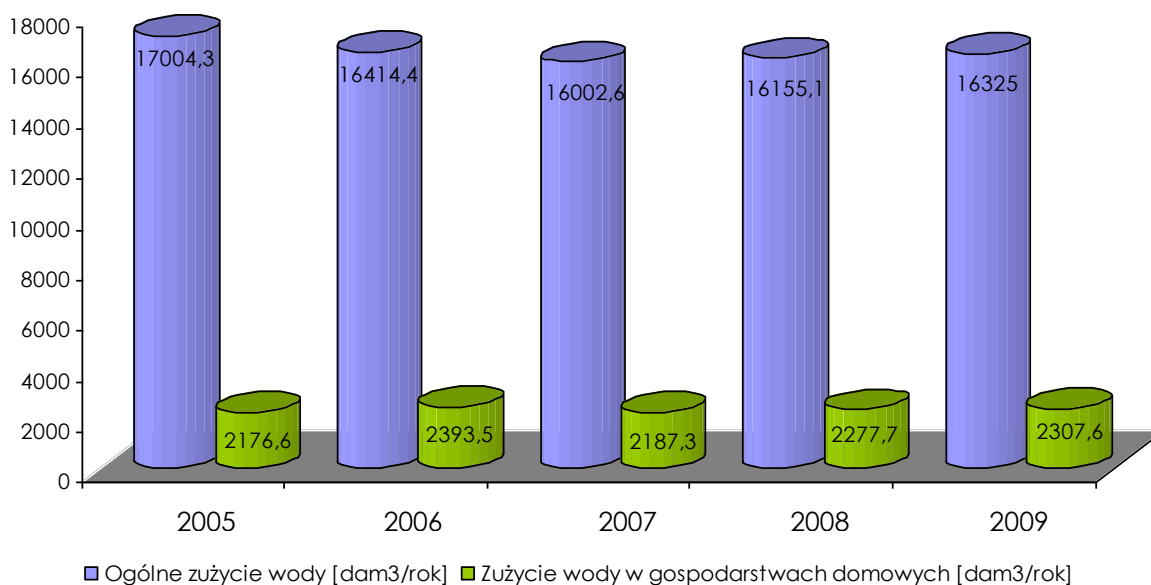
Wykres 6. Zużycie wody w powiecie [tys. m 3 /rok]
